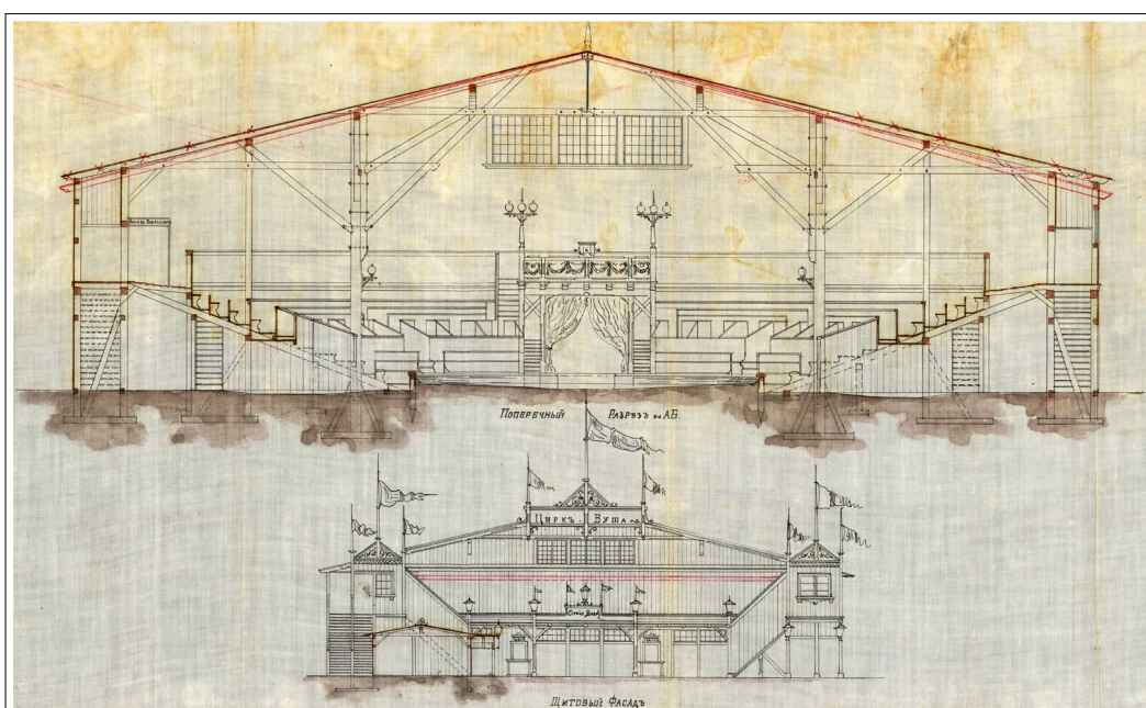
Projekt drewnianego namiotu dla niemieckiego cyrku Paula Buscha u zbiegu ulic Spacerowej, Zielonej i Wólczańskiej (obecnie al. Kościuszki 1 i ul. Wólczańska 18), 1889 r. Rząd Gubernialny Piotrkowski, seria: Wydział Budowlany, sygn. 1082
