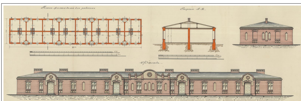
Projekt budowy jednego z dwunastu murowanych, parterowych domów dla robotników Łódzkiej Fabryki Nici na Widzewie, 1908 r. Towarzystwo Akcyjne Łódzkiej Fabryki Nici Spółka Akcyjna Łódź, sygn. 127, nlb.
