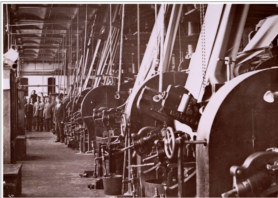
Maszyny do drukowania tkanin w fabryce Izraela K. Poznańskiego przy ul. Ogrodowej. Wg Akcionernej Obszczestwo Bumażnych Manufaktur I.K. Poznanskawo w Lodzi / Société par Actions des Manufactures de Coton J.K. Poznanski Lodz, Łódź 1900. Zbiór albumów ikonograficznych, sygn. A-142, k. 10
