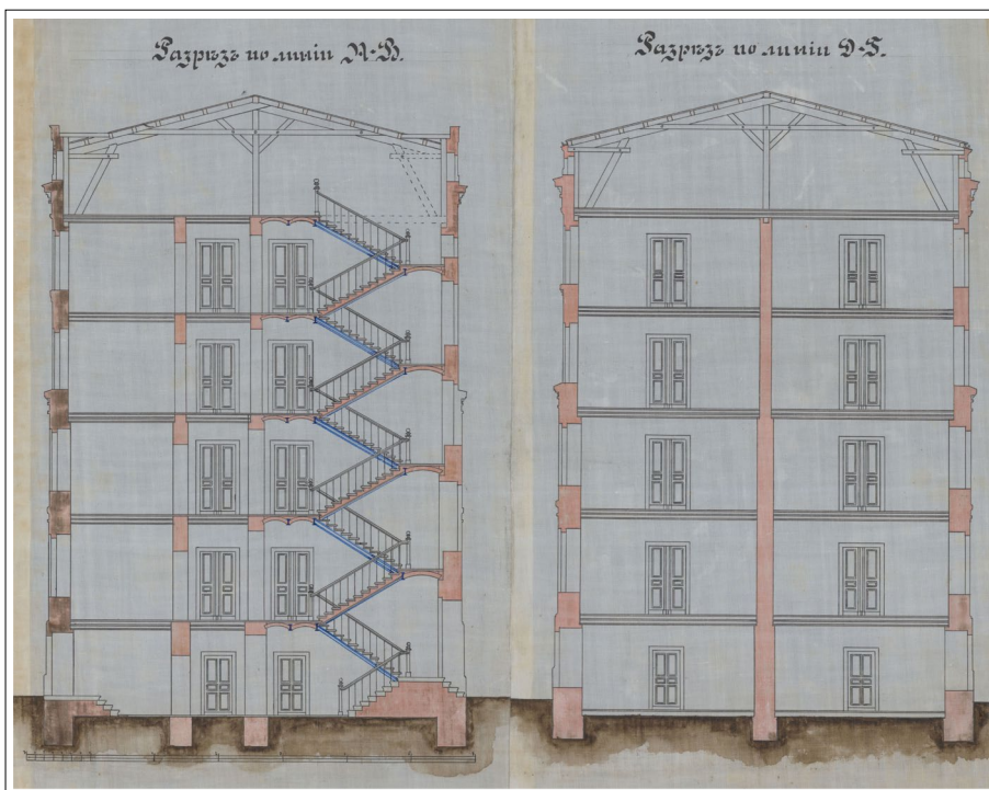
Plan murowanego domu mieszkalnego dla robotników fabrycznych przy ul. Ogrodowej 64 (obecnie ul. Ogrodowa 28). Przekroje poprzeczne. Proj. Franciszek Chełmiński, 1896 r. Rząd Gubernialny Piotrkowski, seria: Wydział Budowlany, sygn. 5775, s. 8
