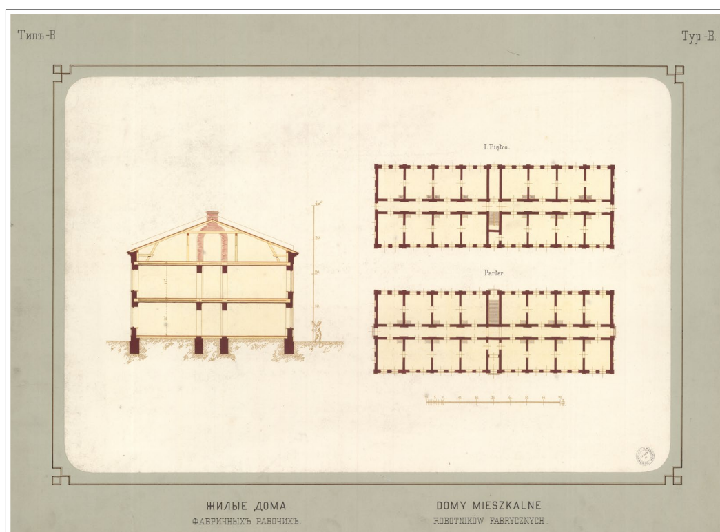
Plan domu w osiedlu robotniczym na Księżym Młynie z 1900 r. Przekrój poprzeczny oraz rzuty poziome parteru i pierwszego piętra. Zbiór kartograficzny Archiwum Państwowego w Łodzi, sygn. 5966
