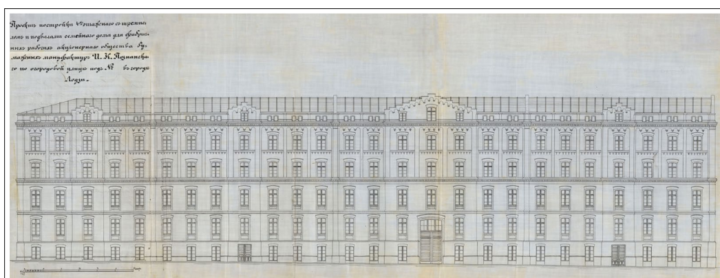
Plan murowanego domu mieszkalnego dla robotników fabrycznych przy ul. Ogrodowej 64 (obecnie ul. Ogrodowa 28). Elewacja frontowa. Proj. Franciszek Chelmiński, 1896 r. Rząd Gubernialny Piotrkowski, seria: Wydział Budowlany, sygn. 5775, s. 8
