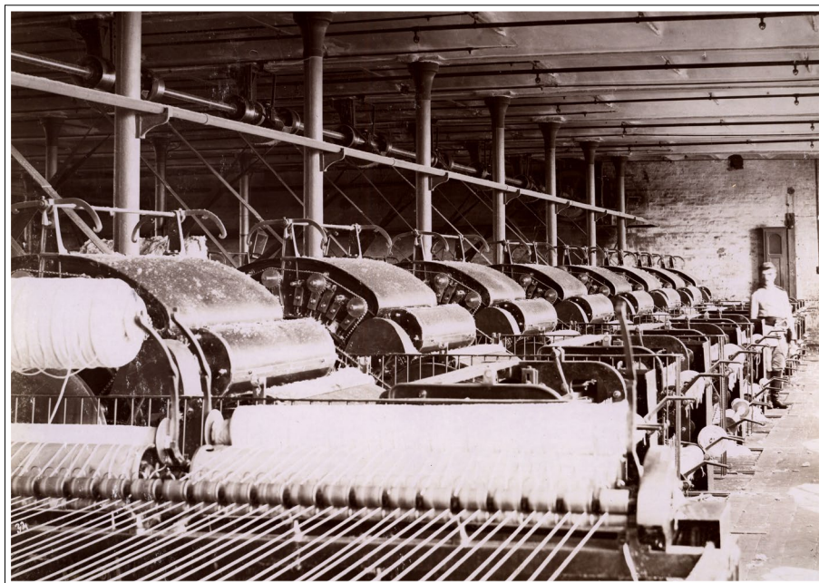
Maszyny do przędzenia odpadów bawełnianych w fabryce Izraela K. Poznańskiego przy ul. Ogrodowej. Wg Aktionernej Obszczestwo Bumażnych Manufaktur I.K. Poznanskawo w Lodzi / Societé par Actions des Manufactures de Coton J.K. Poznanski Lodz , Łódź 1900. Zbiór albumów ikonograficznych, sygn. A-142, k. 3
