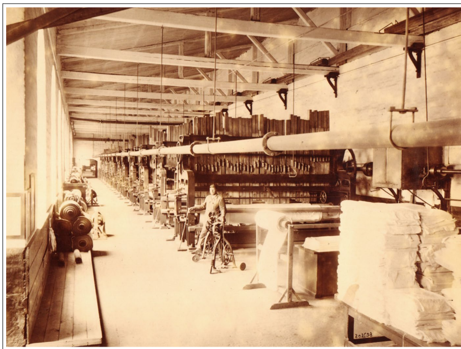
Sala bielnika w zakładach Scheiblerowskich. Fot. Jules David, przełom XIX i XX w. Zbiór ikonograficzny Archiwum Państwowego w Łodzi, seria: Fabryki, podseria: Zjednoczone Zakłady K. Scheiblera i L. Grohmana, sygn. 223
