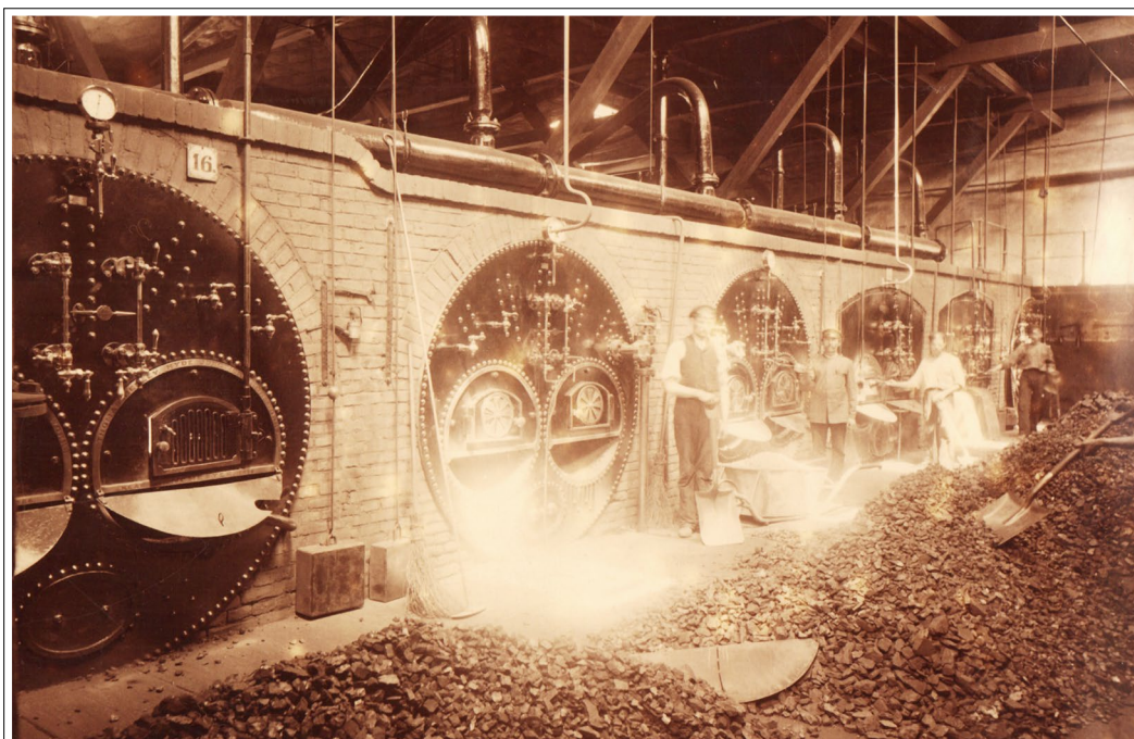
Kotłownia w fabryce na Księżym Młynie. Fot. Jules David, przełom XIX i XX w. Zbiór ikonograficzny Archiwum Państwowego w Łodzi, seria: Fabryki, podseria: Zjednoczone Zakłady K. Scheiblera i L. Grohmana, sygn. 207
