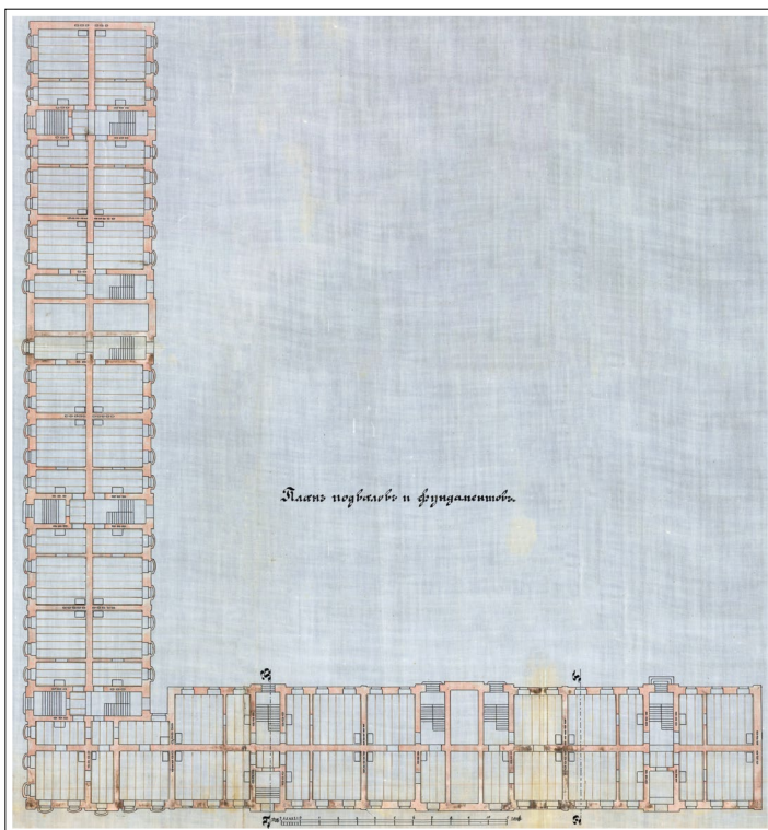
Plan murowanego domu mieszkalnego dla robotników fabrycznych przy ul. Ogrodowej 64 (obecnie ul. Ogrodowa 28). Rzut poziomy. Proj. Franciszek Chełmiński, 1896 r. Rząd Gubernialny Piotrkowski, seria: Wydział Budowlany, sygn. 5775, s. 8
