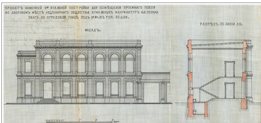
Budynek ambulatorium i poczekalni przy ul. Ogrodowej (obecnie ul. Drewnowska 58b), 1893 r. Rząd Gubernialny Piotrkowski: seria: Wydział Budowlany, sygn. 3258, k. 7
